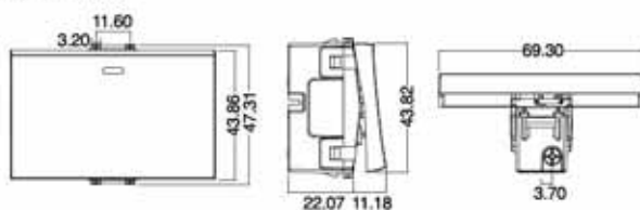
Figure 11 - สวิตช์ขนาดใหญ่
