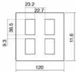
Figure 23 - แผง 4 ช่อง
