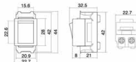
Figure 2 - สวิตช์ 2 ทาง 16A 250V-
