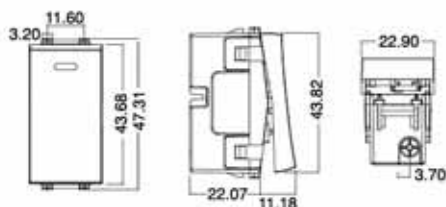
Figure 9 - สวิตช์ขนาดมาตรฐาน
