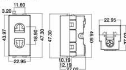
Figure 13 - เต้ารับเดี่ยว 2 ขา
