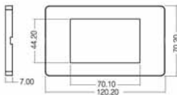
Figure 5 - แผงหน้ากรากพลาสติก 4 ช่อง
