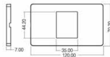
Figure 4 - แผงหน้ากราก 1 ช่องสกรู
