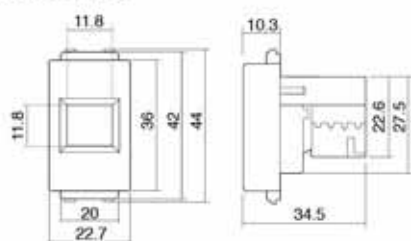
Figure 13 - ตัวรับคอมพิวเตอร์ CAT 5E
