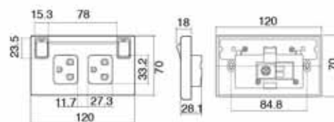
Figure 10 - ตัวรับคู่มีกราวด์ สวิตช์และไฟสัญญาณ
