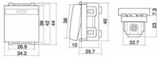
Figure 2 - สวิตช์ 1 ทางขนาดกลาง
