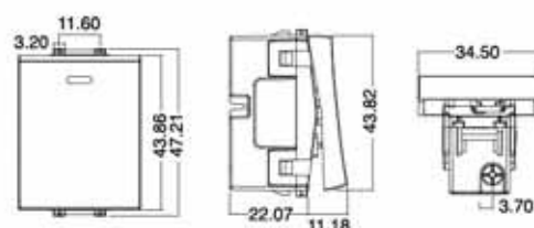
Figure 10 - สวิตช์ขนาดกลาง
