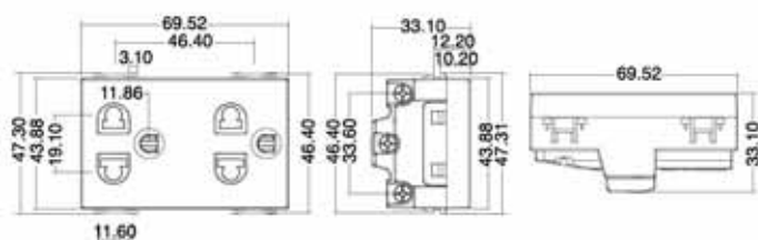
Figure 15 - เต้ารับคู่มีกราวด์ 3 ขา
