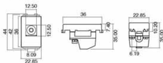
Figure 11 - ตัวรับโทรศัพท์
