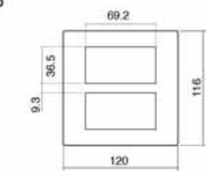
Figure 24 - แผง 6 ช่อง
