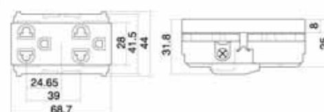
Figure 4 - เต้ารับคู่เสียบขากกลมแบบ มีกราวด์
