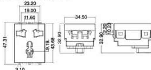
Figure 14 - เต้ารับเดี่ยวมีกราวด์ 3 ขา 18 แบบ
